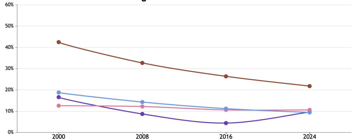
Entwicklung der Indikatorwerte von Mali
