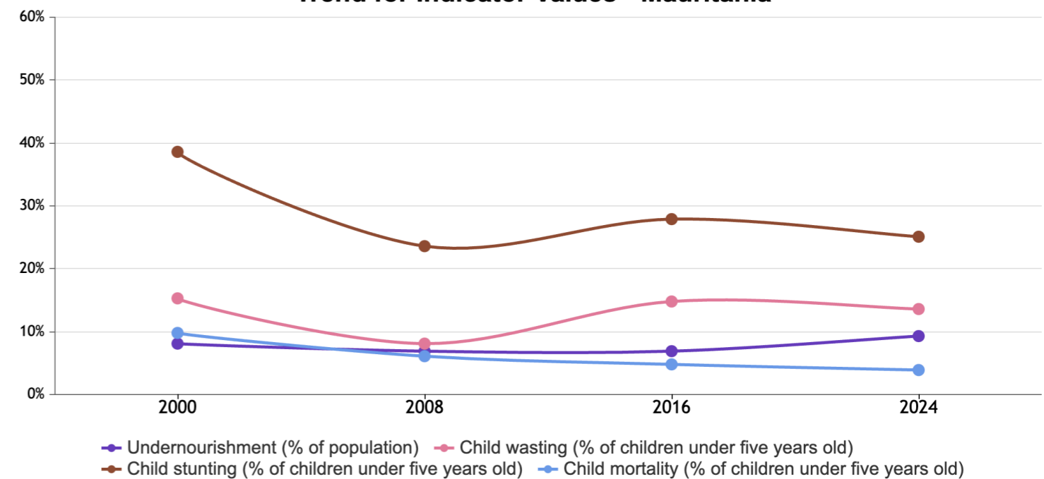
Trend for Indicator Values - Mauritania
